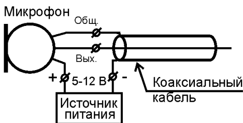
а) подключение к коаксиальному кабелю
