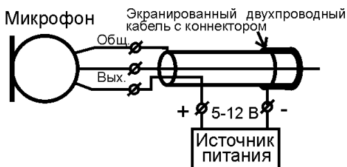
б) подключение к экранированному двухпроводному кабелю
