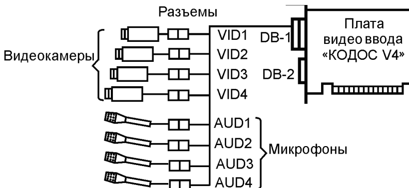
Рисунок 3 – Схема подключения видеокамер и микрофонов
