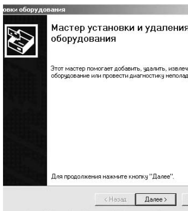
Рисунок А.3 - Окно «Мастер установки и удаления оборудования»
