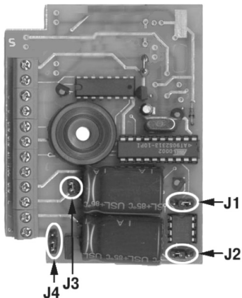
Рисунок 3 – Перемычки контроллера
