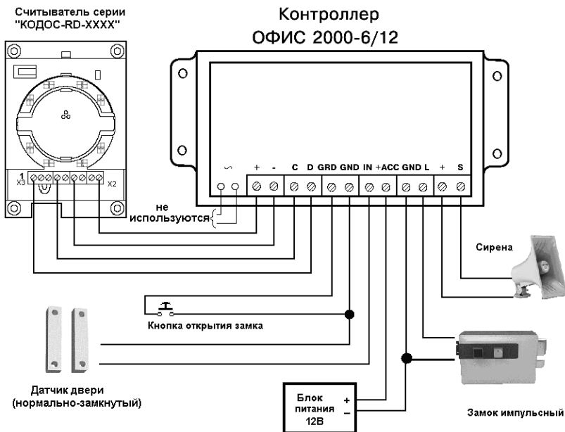
Рисунок 2 – Схема подключения к контроллеру внешних устройств
