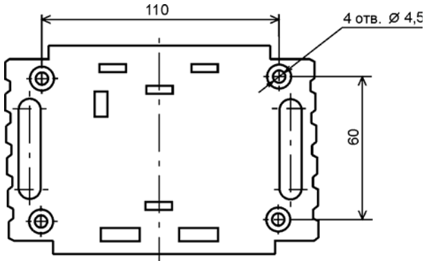
Рисунок 5 -- Крепление изолятора линии (присоединительные размеры)
