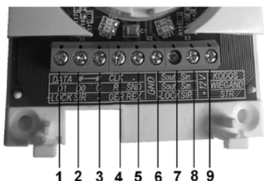
Рисунок 4 – Клеммы считывателя без переключки
