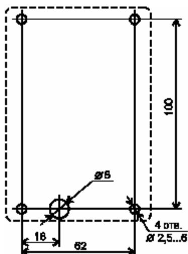
Рисунок 6 – Установочные размеры
