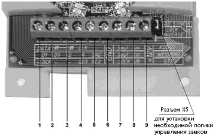
Рисунок 3 – Клеммы контроллера
