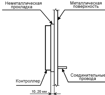
Рисунок 5 – Установка контроллера на металлическую поверхность
